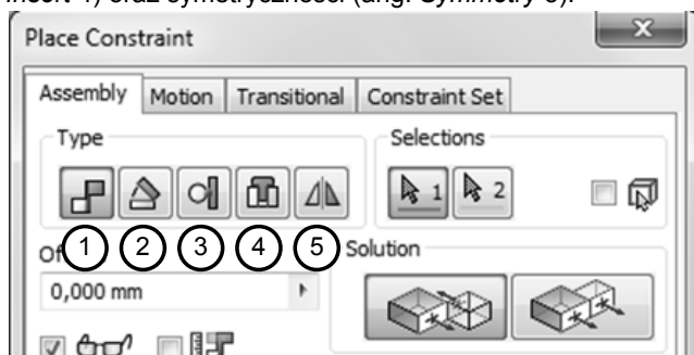
Rys. 2. Przybornik z narzędziami wiązań części i podzespołów, wiązanie: (1) zestawiające, (2) kątowe, (3) styczne, (4) wstawiające, (5) symetryczne
