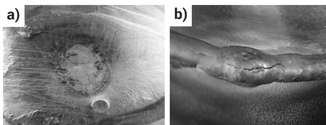
Rys. 2. Niezgodności typu pęknięcia w złączu próbným: a) pęknięcie promieniste, b) pęknięcie w grani spoiny Fig. 2. Welding imperfection in weld specimens: a) radial crack, b) longitudinal crack
