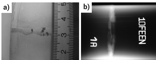
Rys. 3. Niezgodności spawalnicze w złączu próbným: a) por gazowy z pęknięciem, b) pęknięcie w osi spoiny Fig. 3. Welding imperfection in weld specimens: a) radial crack, b) longitudinal crack
