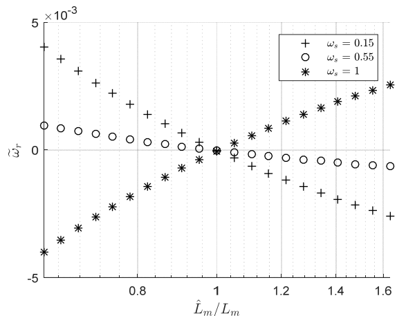
Rys. 9. Błędy odtwarzania prędkości wirnika w funkcji błędu indukcyjności głównej maszyny nieobciążonej
