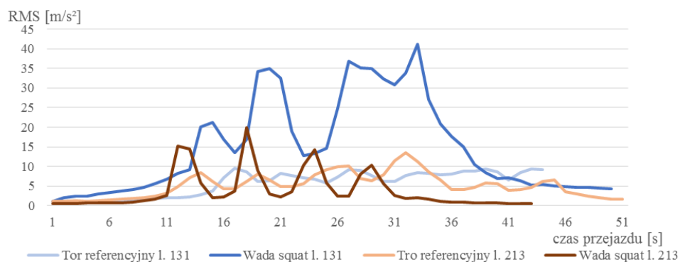
Rys. 6. Wyniki pomiarów z czujnika trójosiowego umiejscowionego na szyjście szyny kierunek Y dla odcinków torów referencyjnych oraz powierzchni z wadą squat
