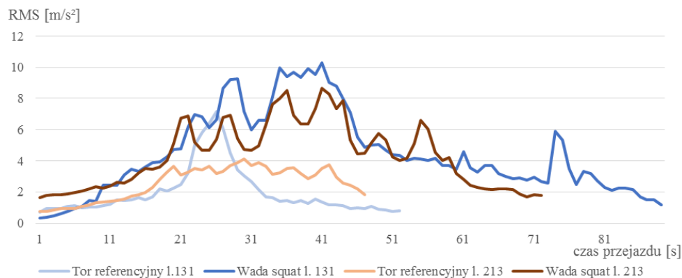
Rys. 5. Wyniki pomiarów z czujnika trójosiowego umiejscowionego na szyjście szyny kierunek X dla odcinków torów referencyjnych oraz powierzchni z wadą squat
