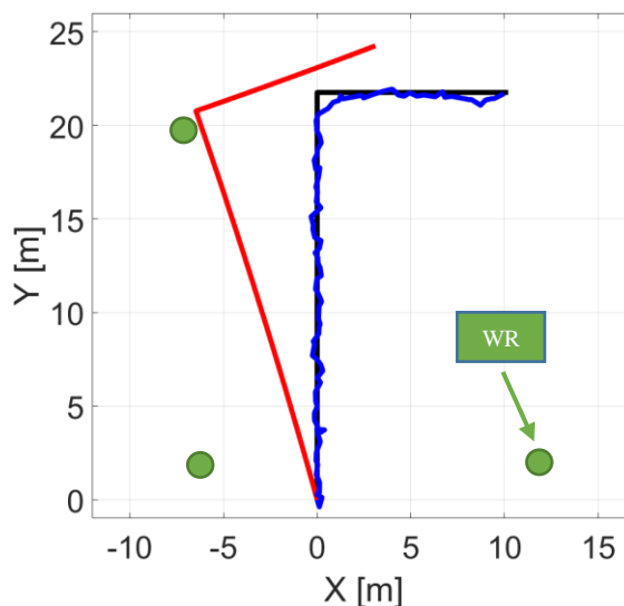
Rys. 4.20. Trasa poruszającej się osoby wyznaczona z użyciem algorytmu nawigacji inercyjnej (kolor czerwony) oraz w procesie integracji danych z użyciem filtracji Kalmana (kolor niebieski) przy dostępnych trzech węzłach referencyjnych o znanym położeniu.
