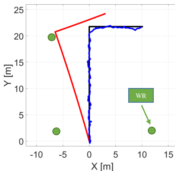
Rys. 4.20. Trasa poruszającej się osoby wyznaczona z użyciem algorytmu nawigacji inercyjnej (kolor czerwony) oraz w procesie integracji danych z użyciem filtracji Kalmana (kolor niebieski) przy dostępnych trzech węzłach referencyjnych o znanym położeniu.
