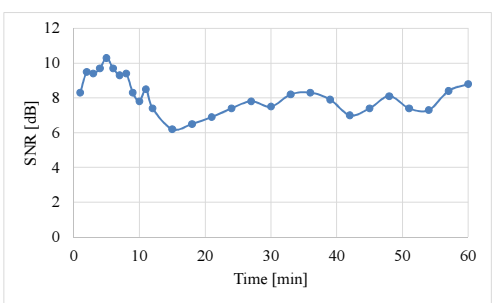
Fig. 9. Multiplex SNR.
