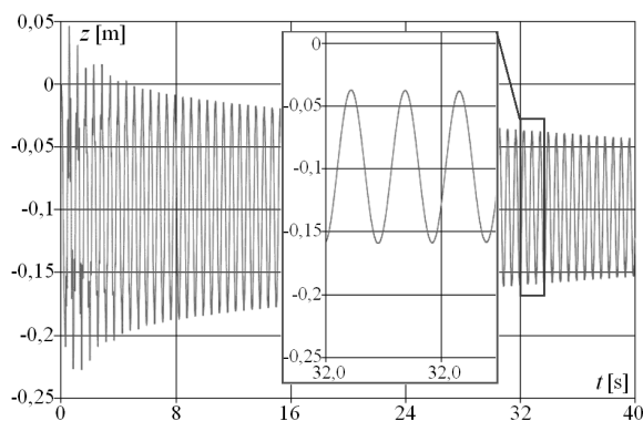
Rys. 5. Wyniki symulacji przebiegu drgań przewodu jezdnego
