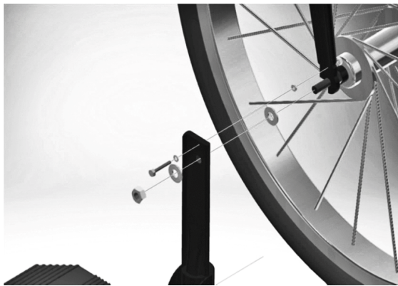
Rys. 5. Wizualizacja łączenia podnóżka z ramą konstrukcyjną Fig. 5. Visualization of connecting the footrest with the construction frame
