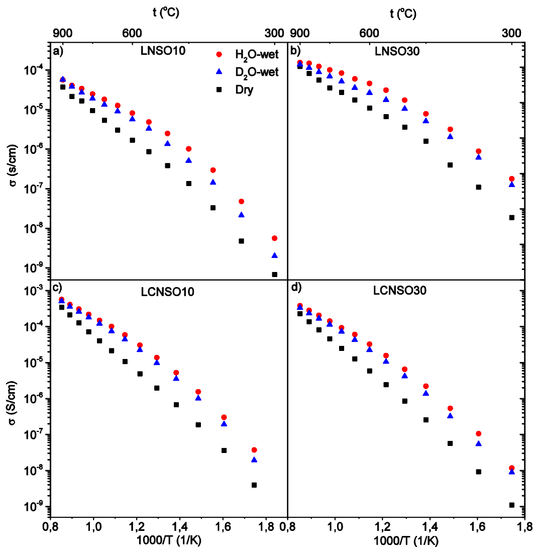
Rysunek 6.21 Przewodność całkowita w funkcji temperatury związku a) LNSO10, b) LNSO30, c) LCNSO10 oraz d) LCNSO30.
