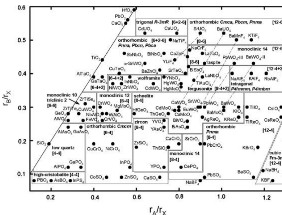
Rysunek 3.3 Diagram Bastide'a z późniejszymi zmianami naniesionymi przez Manjòn i Errandonea 125 .
