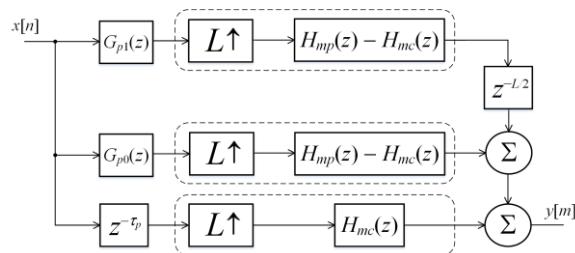
Rys. 7. Schemat interpolatora bazującego na filtrze FRM
