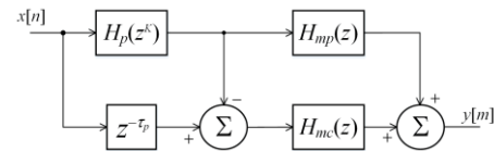
Rys. 2. Struktura filtra FRM
