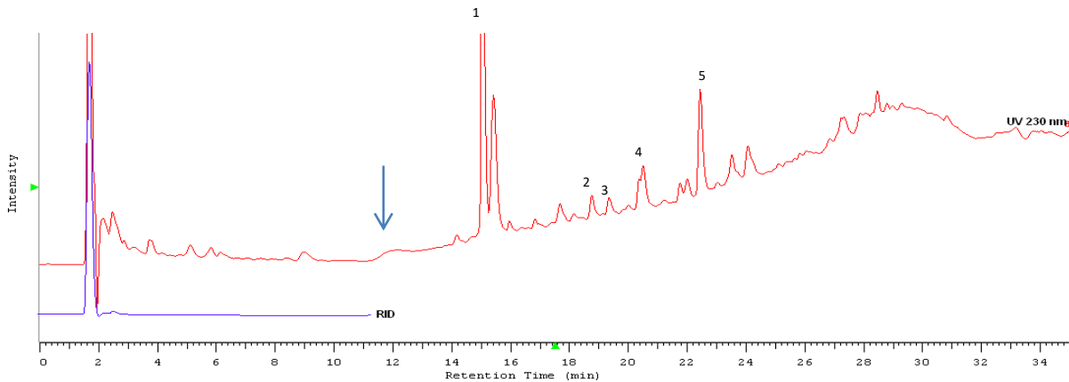
Rys. 34. Nałożone chromatogramy z detektora RID (niebieska linia) oraz UV 230 nm (czerwona linia) - Hydrolyzate 5% NaOH , temp. 90°C, czas: 24 h — objętość dozowana - 50 \mu l, warunki rozdzielania: metoda B , Piki: 1- kwas 4-hydroksybenzoesowy, 2- kwas 3,4-dihydroksybenzoesowy, 3- kwas 4-OH-3,5-metoksybenzoesowy i 4-hydroksy-3-metoksybenzaldehyd, 4-2-metoksyfenol, 5- kwas t-ferulowy, reszta pików niezidentyfikowana-powiększenie Fig. 34. Superimposed chromatograms for detectors: RID (blue line) and UV 230 nm (red line) – hydrolysate 5% NaOH, temp. 90°C, time: 24 h – dosing volume - 50 \mu l, separation condition: method B , Peaks: 1- 4-hydroxybenzoic acid, 2- 3,4-dihydroxybenzoic acid, 3- 4-OH-3,5-methoxybenzoic acid and 4-hydroxy-3-methoxybenzaldehyde, 4-2-methoxyphenol, 5- t-ferulic acid, the rest of peaks are unidentified –enlargement.
