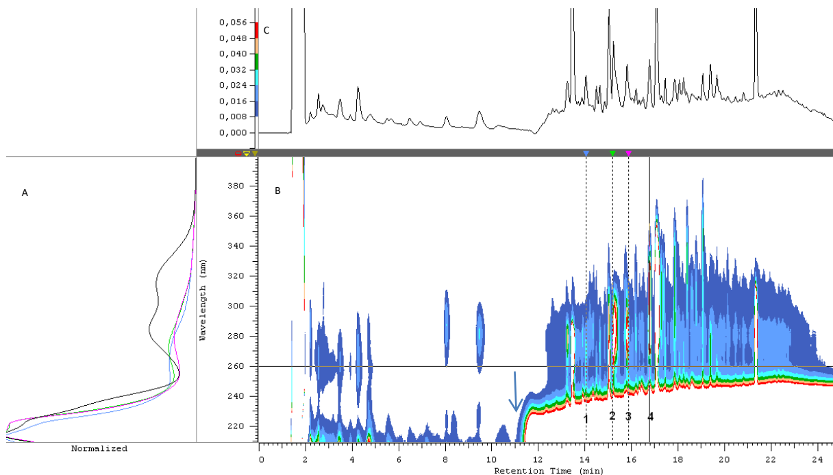
Rys. 18. Chromatogram rozdzielania hydrolizatu wierzby energetycznej, warunki hydrolizy: katalizator: 5% Na 2 CO 3 , temp. 90°C, czas: 24 h, warunki rozdzielania: metoda A, objętość dozowana: 50 µl, A –widma wybranych składników, B – Chromatogram detektora UV-VIS DAD w odwzorowaniu poziomicowym, C -Chromatogram dla 260 nm, Piki: 1 -kwas 4-hydroksybenzoesowy, 2 -kwas 3,4-dihydroksybenzoesowy, 3 -kwas 4-OH-3,5-metoksybenzoesowy, 4 -4-hydroksy-3-metoksybenzaldehyd, reszta pików niezidentyfikowana
