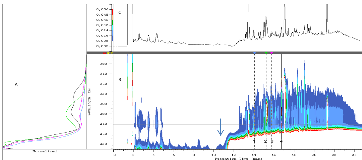
Rys. 17. Chromatogram rozdzielania hydrolizatu wierzby energetycznej, warunki hydrolizy: katalizator: 5% Ca(OH) 2 , temp. 90°C, czas: 24 h, warunki rozdzielania: metoda A, objętość dozowana: 50 µl, A –widma wybranych składników, B – Chromatogram detektora UV-VIS DAD w odwzorowaniu poziomicowym, C -Chromatogram dla 260 nm, Piki: 1 -kwas 4-hydroksybenzoesowy, 2 -kwas 3,4-dihydroksybenzoesowy, 3 -kwas 4-OH-3,5-metoksybenzoesowy, 4 -4-hydroksy-3-metoksybenzaldehyd, reszta pików niezidentyfikowana
