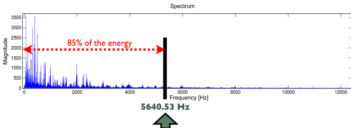
Fig. 6. Roll-off parameter illustration (MIRtoolbox).
