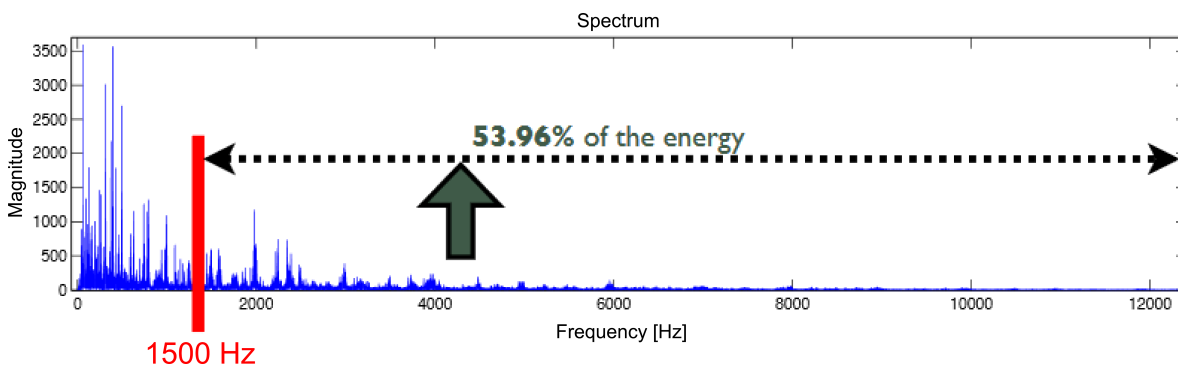
Fig. 3. Brightness (MIRtoolbox).
