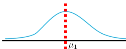
Fig. 2. Centroid (MIRtoolbox).
