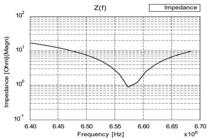
Rys. 3.2. Przykładowa charakterystyka impedancyjna emitera HVR z czasą paraboloidalną (rys. 2.3). Częstotliwość rezonansu własnego – 6,58 MHz
