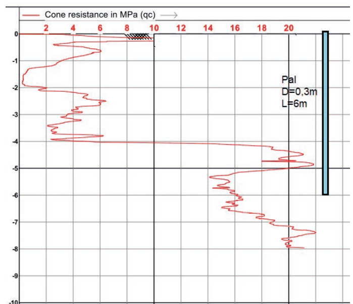
Rys. 4. Sondowanie CPT4
