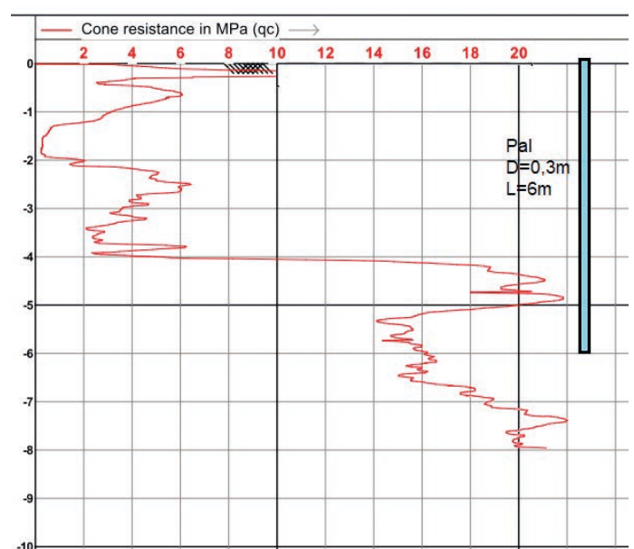
Rys. 4. Sondowanie CPT4
