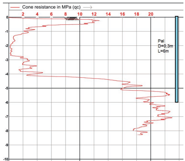
Rys. 3. Sondowanie CPT3
