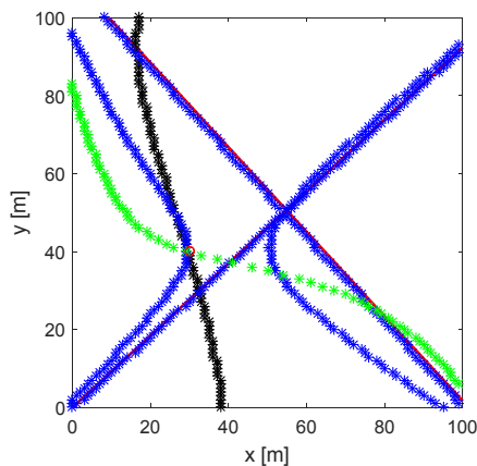
Rys. 3.8. Miejsca zerowe macierzy Vx liczone względem kolumn.
