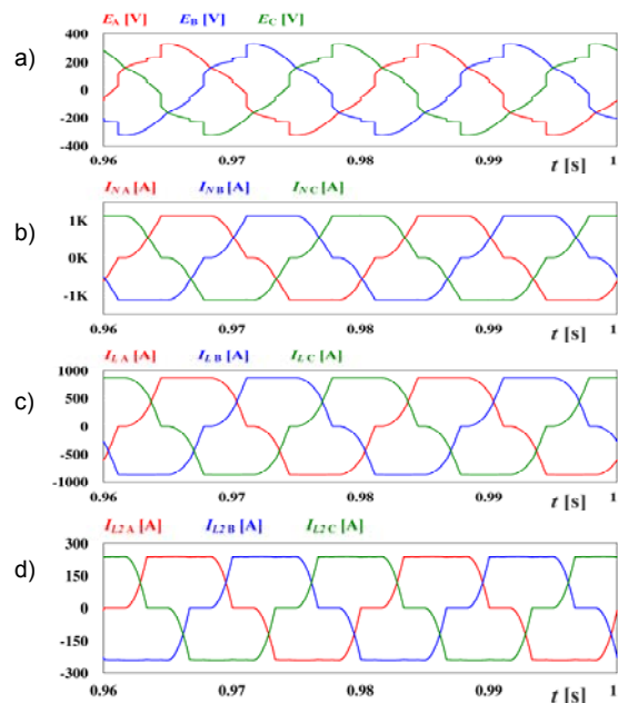
Rys. 7. Przebiegi czasowe prądów i napięć w sieci rozgałęzianej, bez filtra aktywnego: a) napięcie sieci; b) prąd sieci; c) prąd obciążenia NL2 włączony w PCC; d) prąd obciążenia NL2 włączony przed PCC
