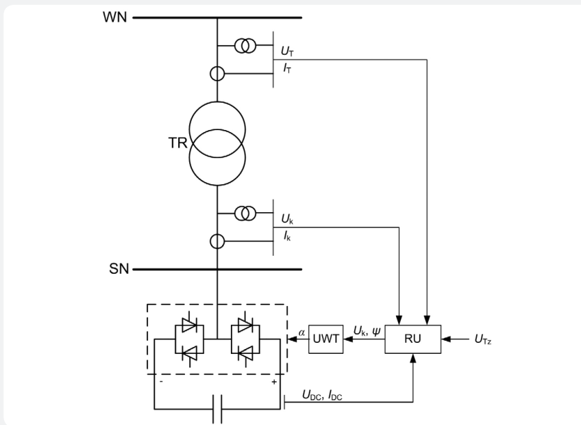
Rys. 2. Struktura układu STATCOM: TR – transformator WN/SN, RU – regulator napięcia, UWT – układysterowania tyrystorów, \alpha – sygnałysterowania przełącznika, U_{Tz} – napięcie zadane, U_T – napięcie kontrolowane, I_T – prąd kompensatora, U_k – napięcie przełącznika, I_k – prąd przełącznika, U_{DC} – napięcie w obwodzie DC, I_{DC} – prąd w obwodzie DC
