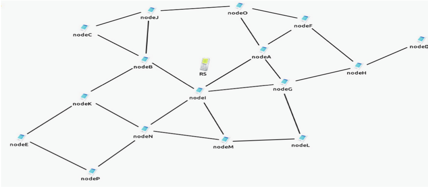
Fig. 7. Simulated 16-node WAHN.
