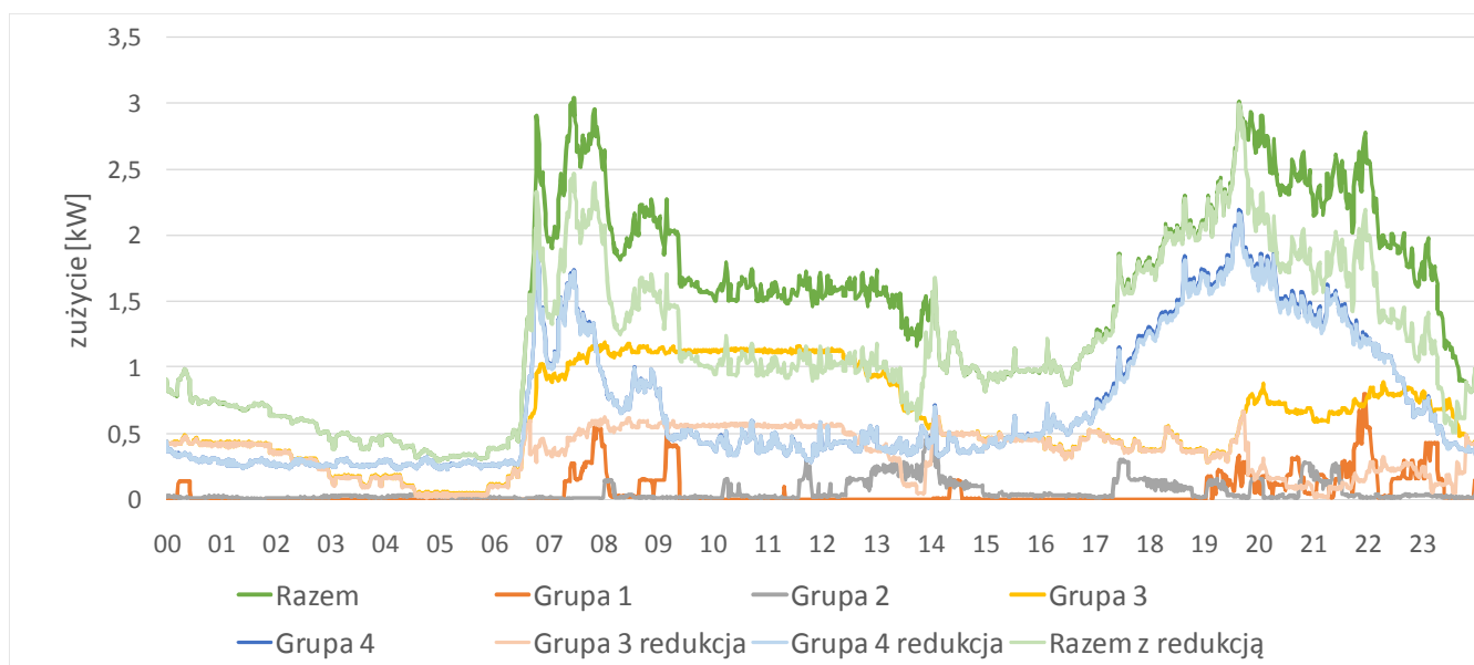
Rys. 3. Średnia dobę roboczą stycznia 2010 – dobowe zapotrzebowanie na moc z uwzględnieniem redukcji zapotrzebowania
