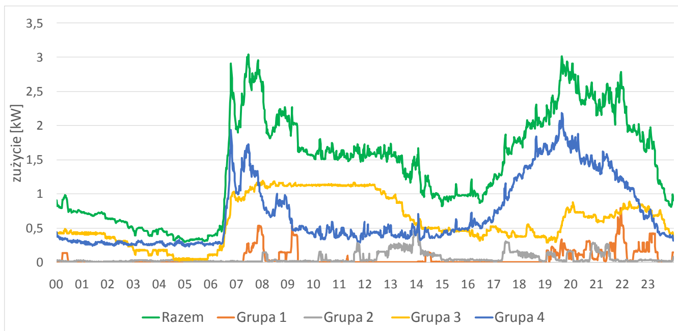
Rys. 2. Średnia dobę roboczą stycznia 2010 – dobowe zapotrzebowanie na moc
