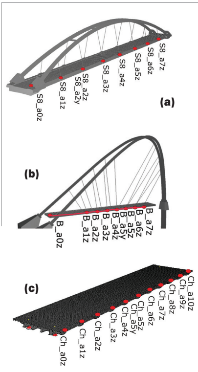
Rys. 8. Rozmieszczenie punktów pomiarowych na kładce (a) nad drogą S8 (b) nad Trasą Uniwersytecką w Bydgoszczy (c) nad ulicą Chwarznieńską w Gdyni
