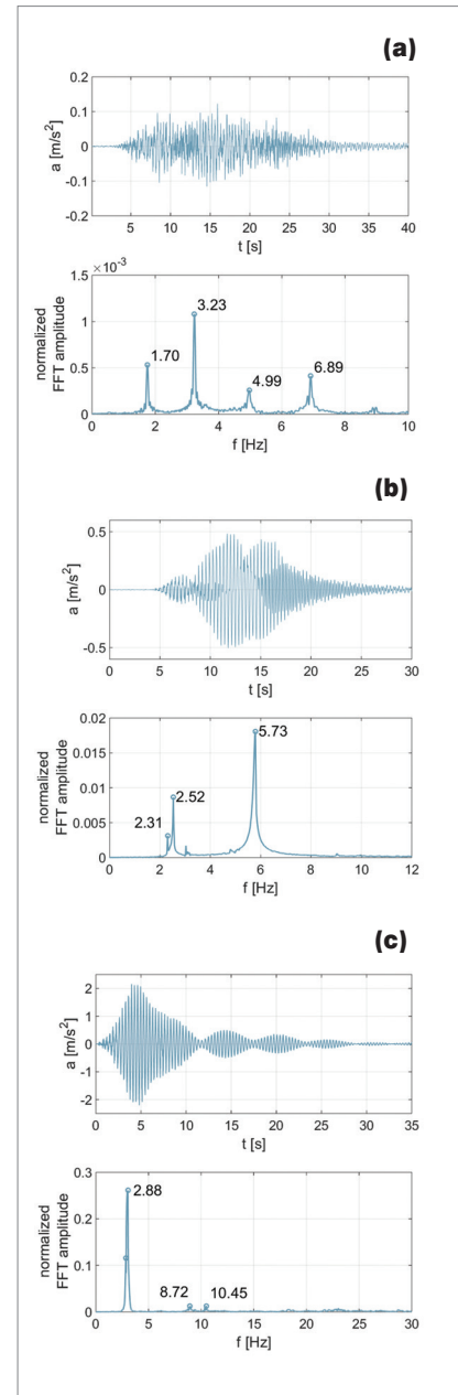
Rys. 9. Reprezentatywne przebiegi przyspieszeń wraz z odpowiadającymi im transformacjami Fouriera dla kładki (a) nad drogą S8 w punkcie a5z od wymuszenia biegiem swobodnym grupy 12 osób (b) nad Trasą Uniwersytecką w Bydgoszczy w punkcie a1z od biegu synchronicznego grupy 9 osób (c) nad ulicą Chwarznieńską w Gdyni w punkcie a5z od wymuszenia marszem synchronicznym grupy 3 osób
