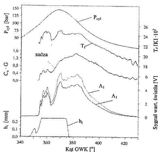
Rys. 5. Temperatura płomienia:
