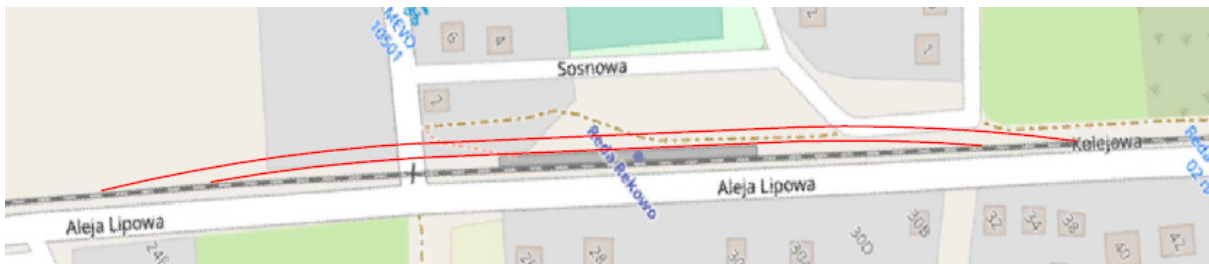
Fig. 3. Proposed location of a staggered track at the Reda Rekowo stop (own elaboration) Rys. 3. Proponowana lokalizacji mijanki na przystanku Reda Rekowo (opracowanie własne)
