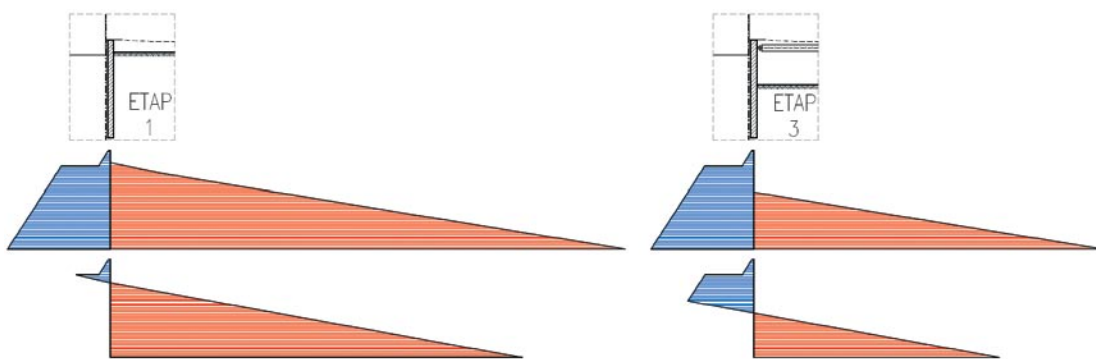
Rys. 5. Schematy występujących oddziaływań na konstrukcję – parcie czynne (kolor niebieski) i parcie bierne/odpór (kolor czerwony)
