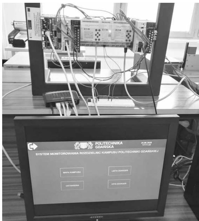
Rys. 8. Stanowisko testowe
