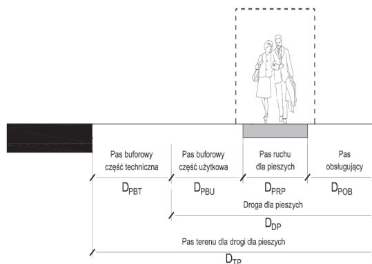
Rys. 16. Schemat przekroju poprzecznego drogi dla pieszych uwzględniający pas terenu przy drodze niezbędny do wybudowania drogi dla pieszych w obszarze zamiejscowym Źródło: opracowanie własne
