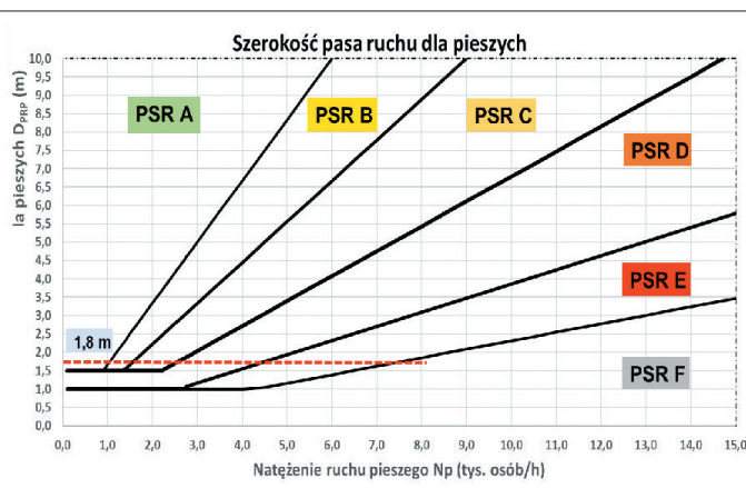
Rys. 21. Pas ruchu dla pieszych – wykres służący do ustalania szerokości pasa w zależności od natężenia ruchu pieszego i przyjętego poziomu warunków ruchu pieszego
