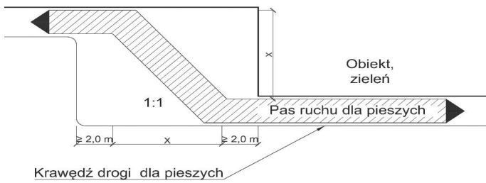
Rys. 22. Schemat placu do zmiany przebiegu pasa ruchu lub drogi dla pieszych w miejscu załamania lub uskoku trasy Źródło: opracowanie własne
