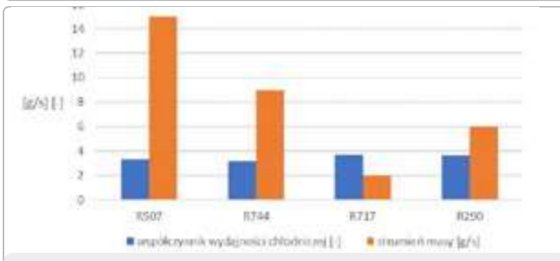
Rys. 18. Porównanie obliczonych wartości wydajności chłodniczej oraz strumienia masy dla grupy specjalnej w zależności od zastosowanego czynnika
