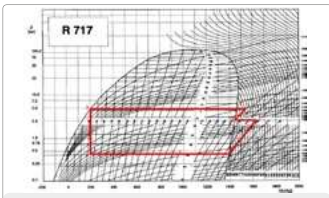
Rys. 11. Przemiany w układzie p-h realizowane w układzie chłodniczym należącym do grupy specjalnej z zastosowaniem R717 jako czynnika roboczego [18]
