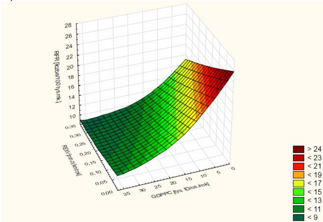
Rys. 6.4 Wpływ wydatków na drogi wojewódzkie REXV oraz jednostkowego produktu krajowego brutto w przeliczeniu na mieszkańca GDPPC na względny wskaźnik ofiar śmiertelnych w wypadkach RFR. Model RFR_PL_07_K3.
