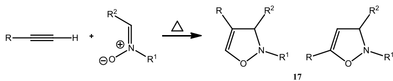
Schemat 8. Reakcja cykloaddycji nitronów z alkinami.
