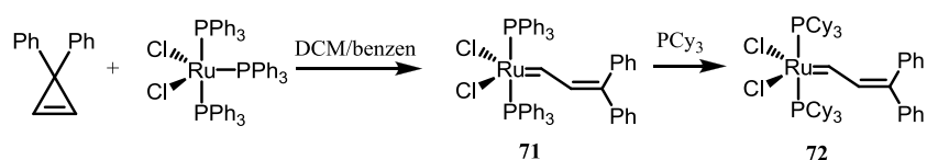
Schemat 39. Pierwsze rutenowe kompleksy alkilidennowe.
