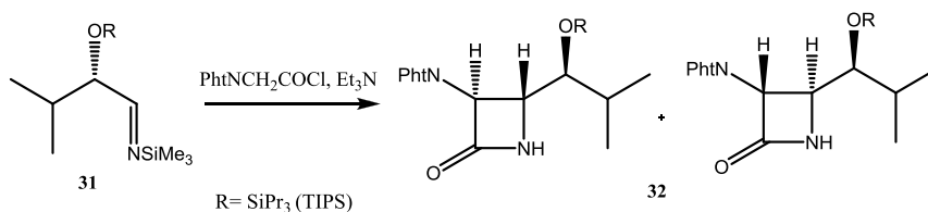
Schemat 19. Asymetryczna synteza trans β-laktamów zawierających chiralny fragment w części aldehydowej iminy.
