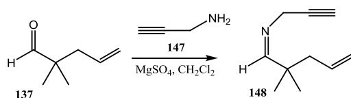
Schemat 92. Synteza iminy 148 zawierającej wiązanie potrójne w części aminowej.
