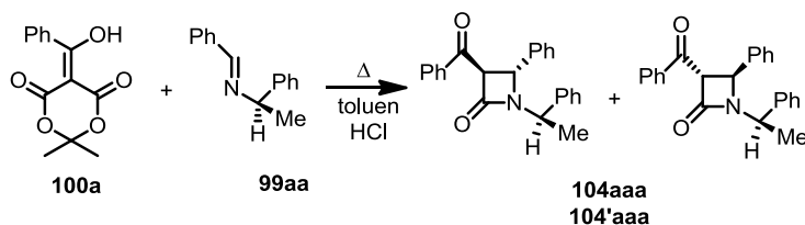
Schemat 63. Reakcja 5-(hydroksy(fenilo)metyleno)-2,2-dimetylo-1,3-dioksa-4,6-dionu 100a z ( R )- N -benzylideno-1-fenyletyloaminą 99aa
