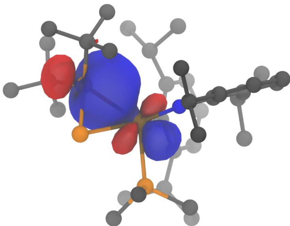
Rysunek 128. Wizualizacja NBO odpowiadającego \sigma(P\beta W) w związku DFT-9.
