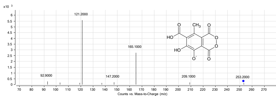
Rysunek S. 75. Produkt fotodegradacji K2 (m/z 253).
