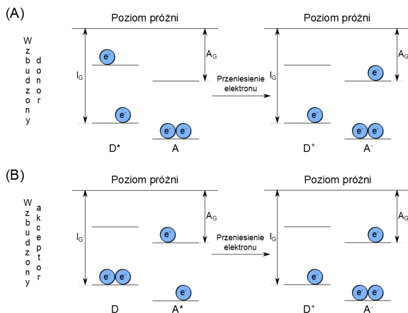
Rysunek 2.6: Mechanizmy powstawania ekscypleksu, gdy wzbudzenie znajduje się na molekuule donorowej (A) i gdy wzbudzona jest molekuła akceptora (B) [6]
