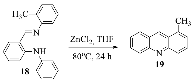
Schemat 4. Synteza pochodnych akrydyny ( 19 ) oparta na reakcji cyklizacji zasady Schiffa o -aryloaminofenyłu w obecności \text{ZnCl}_2 [11].
