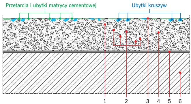
RYS. 4. Etap III degradacji posadzki lastrico; rys.: autorzy 1 – matryca cementowa, 2 – kruszywa różnych gradacji, 3 – impregnat, 4 – lastrico, 5 – mostek szpepny, 6 – podkład betonowy
