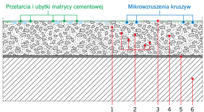
RYS. 3. Etap II degradacji posadzki lastrico; rys.: autorzy 1 – matryca cementowa, 2 – kruszywa różnych gradacji, 3 – impregnat, 4 – lastrico, 5 – mostek szpepny, 6 – podkład betonowy
