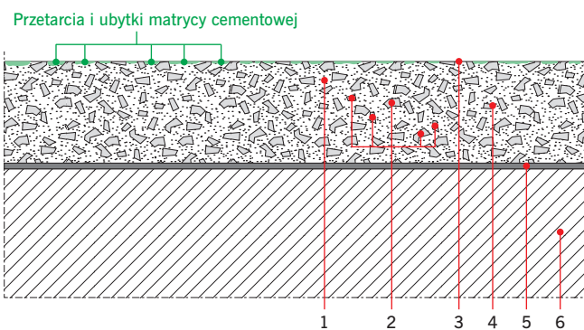
RYS. 2. Etap I degradacji posadzki lastrico; rys.: autorzy 1 – matryca cementowa, 2 – kruszywa różnych gradacji, 3 – impregnat, 4 – lastrico, 5 – mostek szpepny, 6 – podkład betonowy
