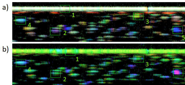
Rys. 6.14. Obraz S-OCTmatrycy PMMA wypełnionej nanocząstkami ditlenku tytanu w trójpas-mowym (a) i jednopasmowym (b) kontraście spektroskopowym uzyskanymi za pomocą algo-rytmu TDR.
