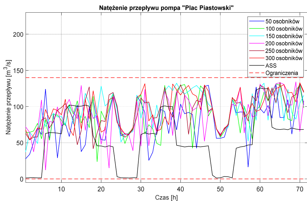
Rysunek 4.37 Porównanie natężenia przepływu dla różnej liczby osobników oraz ASS dla PSSW Chojnice na horyzoncie czasu od 1 do 72 [h], dla pompy „Plac Piastowski”.
