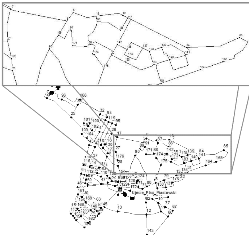
Rysunek Z1.12 Struktura PSSW Chojnice z zaznaczonymi nazwami rurowciągów
