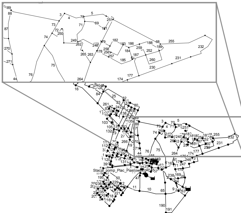
Rysunek Z.4 Struktura PSSW Chojnice z zaznaczonymi nazwami rurociągów.
