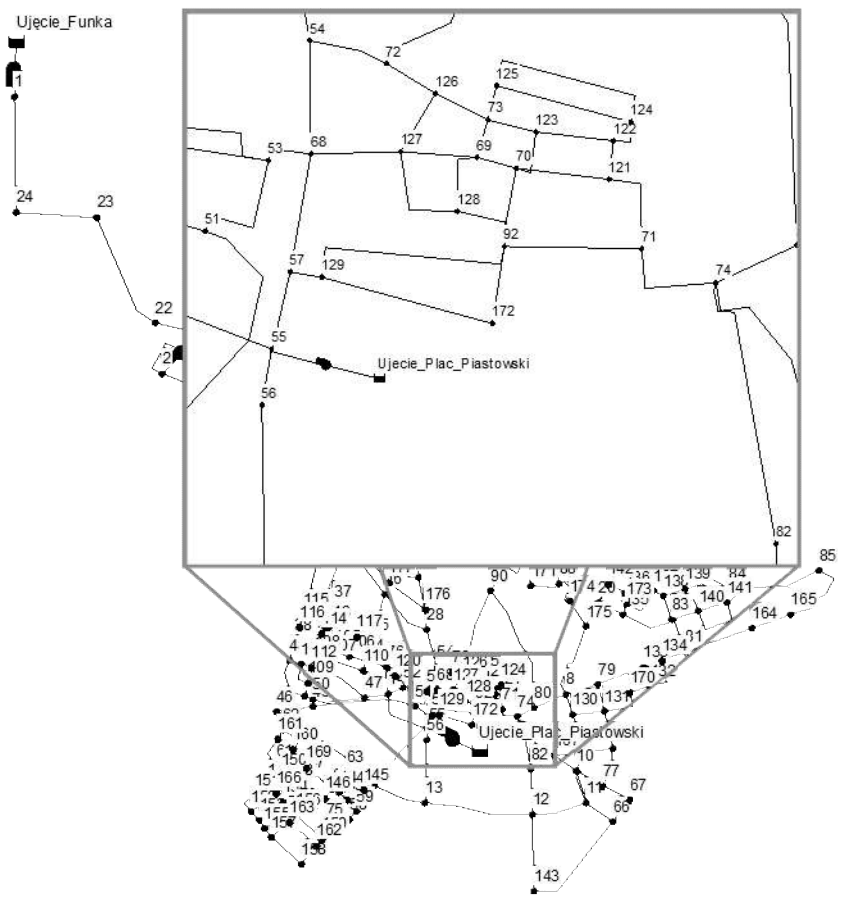
Rysunek Z1.16 Struktura PSSW Chojnice z zaznaczonymi nazwami rurociągów.
