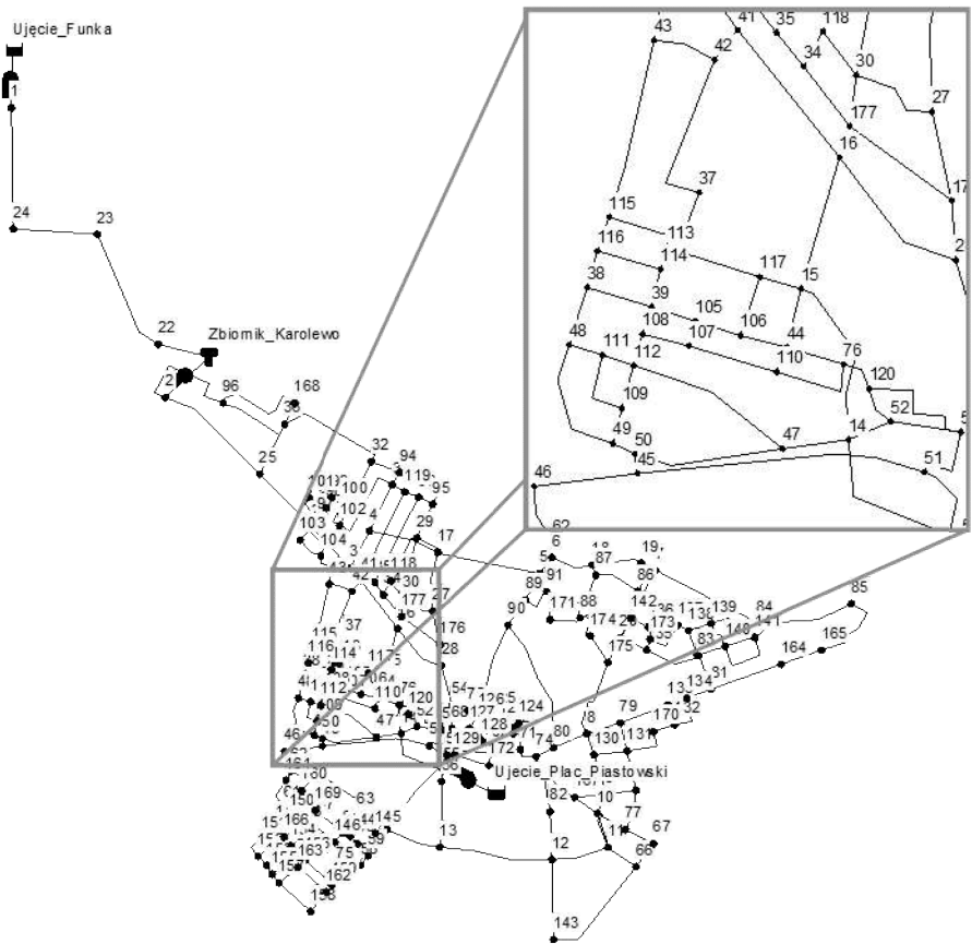
Rysunek Z1.15 Struktura PSSW Chojnice z zaznaczonymi nazwami rurociągów.
