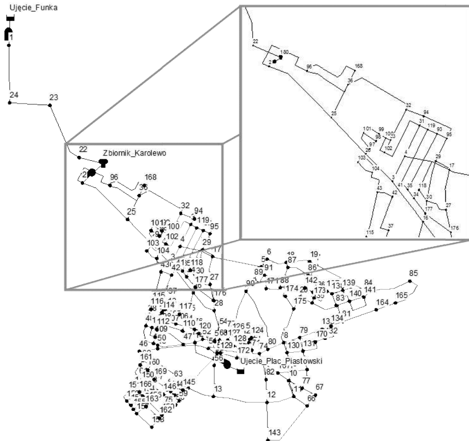
Rysunek Z1.11 Struktura PSSW Chojnice z zaznaczonymi nazwami rurowciągów.
