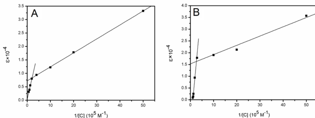
Rys.94. Wykres zależności współczynnika ekstynkcji od odwrotności stężenia przy \lambda = 409 nm dla koniugatów K-Amb-4 (A) i K-Amb-6 (B).
