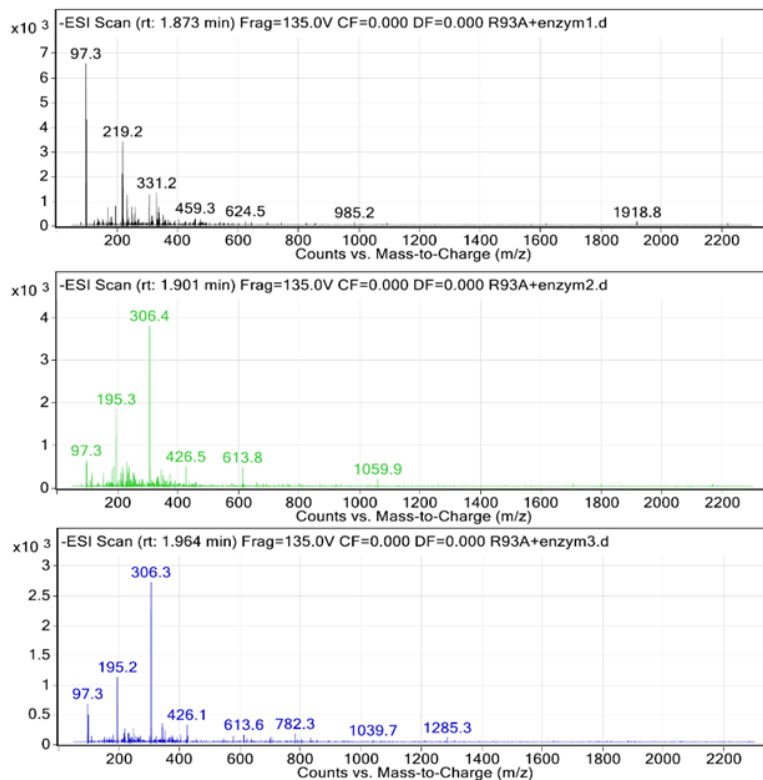
Rys.65. Widma masowe związku K-Umb-11, który został poddany działaniu esterazy (czas trwania hydrolizy: 0, 40 i 120 minut).
