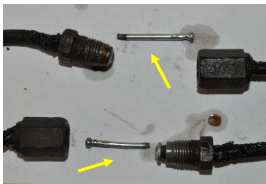
Rys. 4.95. Fragmenty rozłączonych przewodów, w których znajdowały się aluminiowe nit
