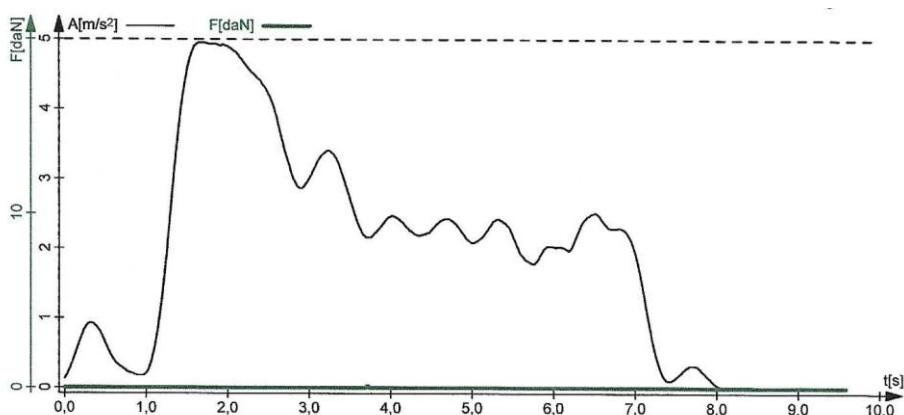
Rys. 8.13. Przebieg opóźnienia hamowania samochodu na mokrej nawierzchni gruntowej z niesprawnym układem ABS - pomiar 8.21
