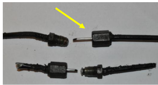
Rys. 4.94. Fragmenty rozłączonych przewodów, w których znajdują się aluminiowe nit
