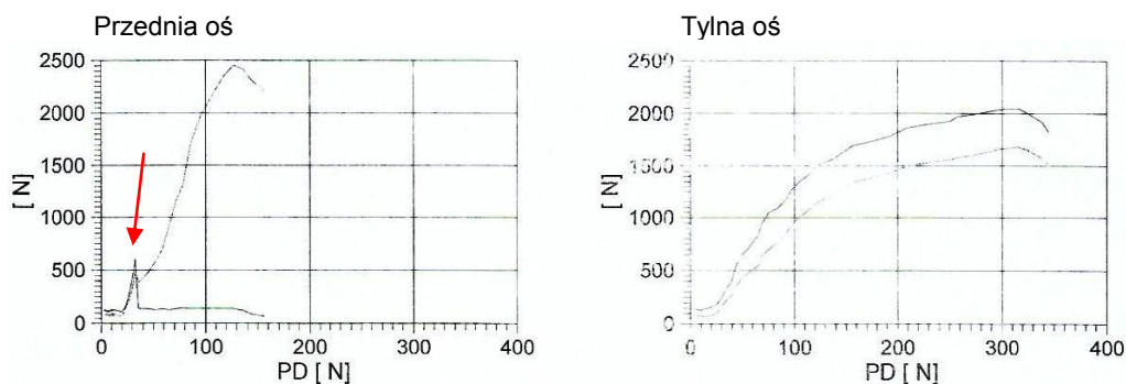
Rys. 6.10. Wykresy zmierzonych sił hamowania samochodu z niesprawnym układem hamulcowym i włączonym ABS (czerwoną strzałką zaznaczono rozszczelnienie układu i wyciek płynu hamulcowego)
