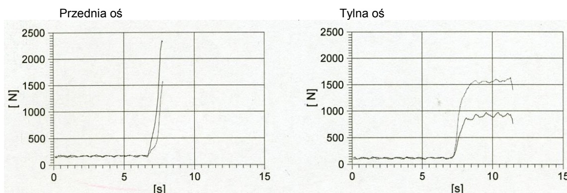
Rys. 5.2. Wykresy zmierzonych sił hamowania samochodu Daewoo Lanos, rok produkcji 2001
