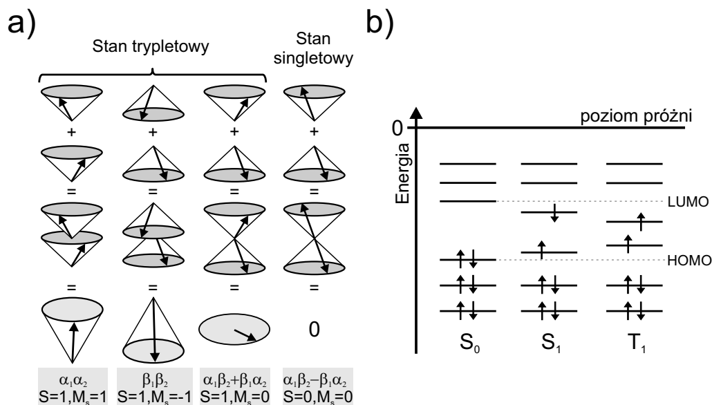
Rysunek 2.2.1. Możliwe konfiguracje wektorowe spinowego momentu pędu (a). Schemat poziomów energii dla stanów singletowych ( S_0, S_1 ) oraz dla stanu trypletowego ( T_1 ). Strzałki oznaczają spiny elektronów (b)
