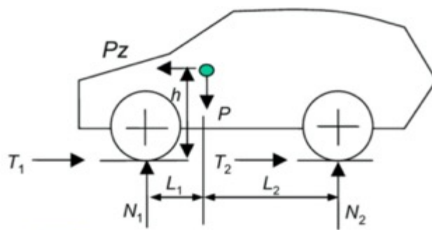
Rys. 8.17. Dwuwymiarowy model pojazdu z rozkładem nacisków kół podczas hamowania czterema kołami [2]
