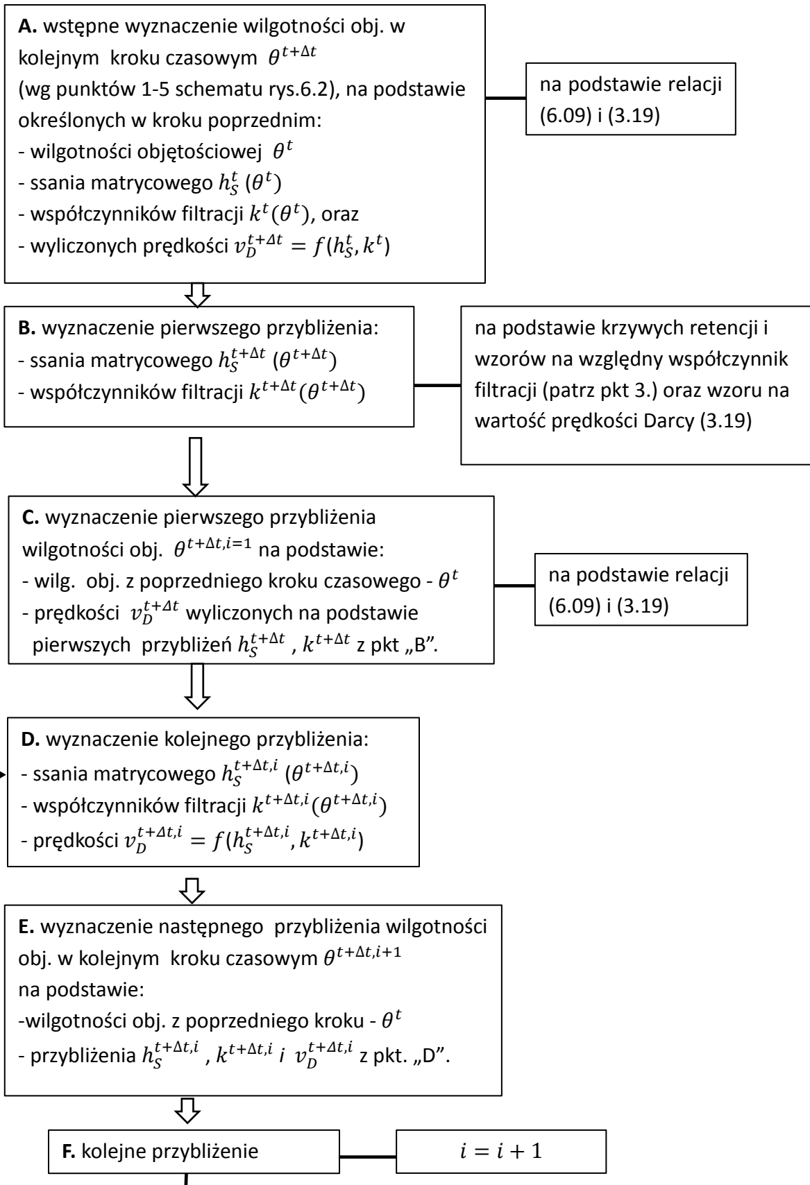
Rys. 6.3. Schemat blokowy wyliczeń wilgotności obj. dla kolejnego kroku czasowego
