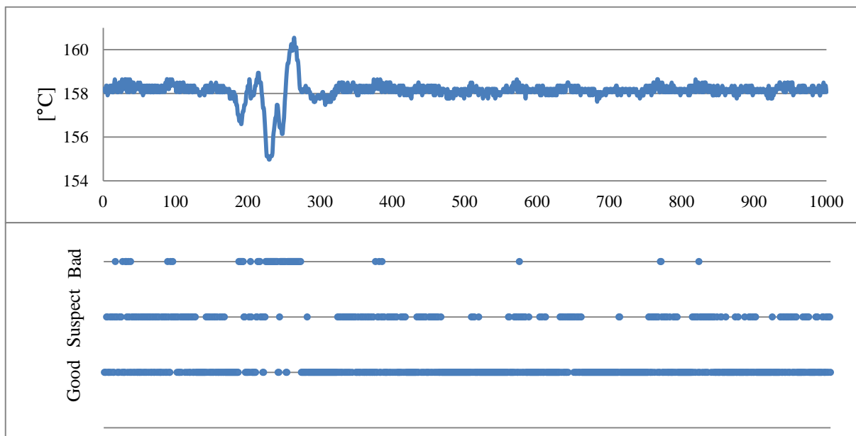
Rys. 5.25 Wykres przedstawiający wartość oraz ocenę dla temperatury kondensatu na wylocie z wymiennika XN4 w przypadku pracy w stanie ustalonym, w którym wystąpiły chwilowe zakłócenia (Wariant II)
