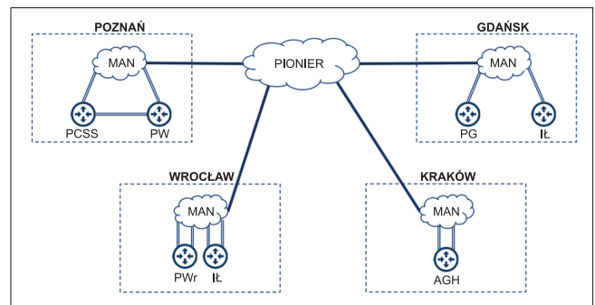
■ Rys. 8. Topologia sieci operacyjnej
