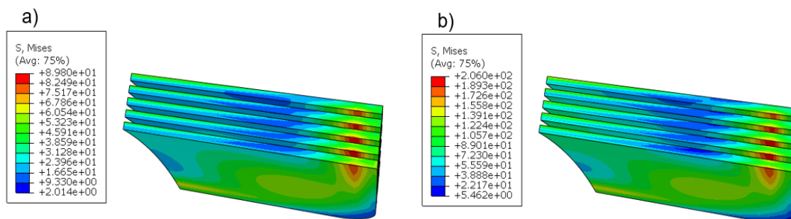
Rys. 163. Mapa naprężeń w szkłe (model 6) dla obciążenia: a) 0,5 MPa; b) 1,0 MPa
