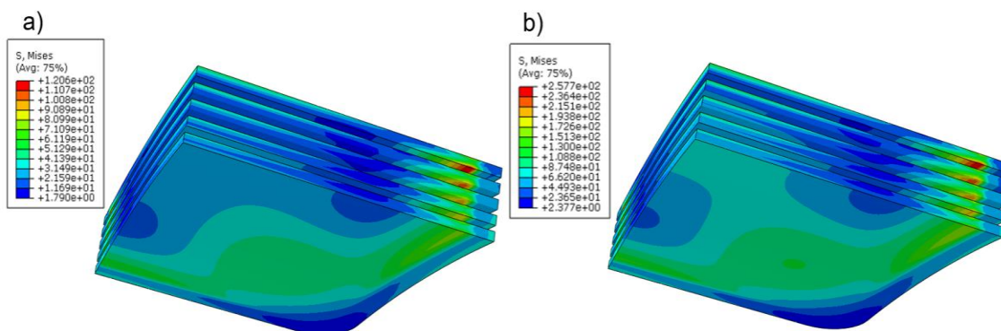
Rys. 161. Mapa naprężeń w szkłe (model 5) dla obciążenia: a) 0,5 MPa; b) 1,0 MPa
