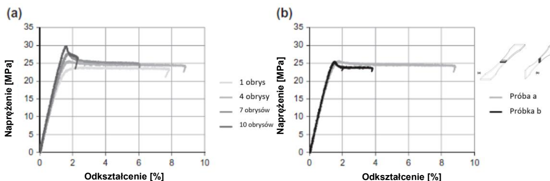
Rys. 17. Krzywe rozciągania napężenie – odształcenie otrzymane podczas statycznej próby rozciągania jednoosiowego z uwzględnieniem: a) różnej liczby obrysów; b) ułożenia próbki - źródło [21]
