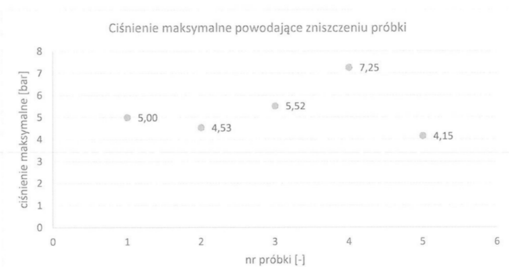
Rys. 131. Wykres ciśnienia maksymalnego powodującego zniszczenie próbki okrągłej - źródło [50]
