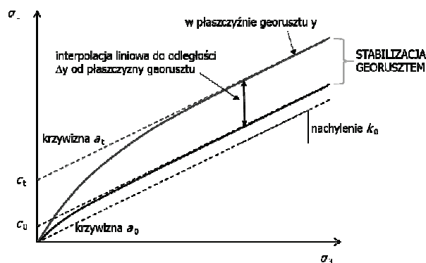
2. Obwiednia zniszczenia kruszywa stabilizowanego georusztem trójosiowym [7]
