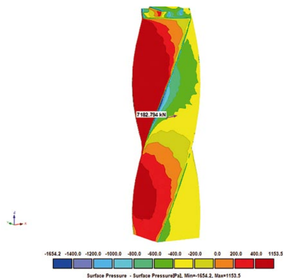
Rys. 9. Rozkład ciśnienia na powierzchni konstrukcji wraz z wypadkową siłą oddziałującą na budynek
