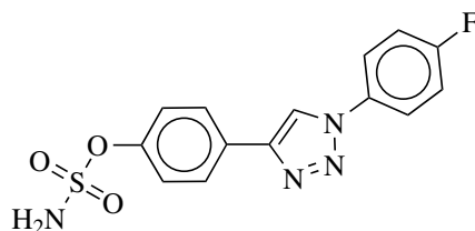
Amidosiarczan 4-(1-(4-fluorofenilo)-1 H -1,2,3-triazol-4-ilo)fenylu Ib
