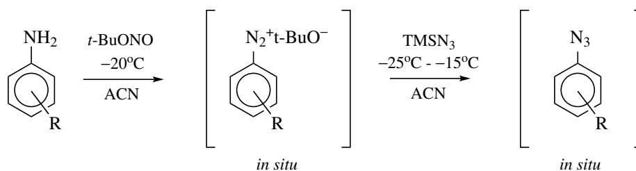
Schemat 2.2: Schemat reakcji optymalizacji otrzymywania pochodnych azydków fenolowych in situ (R = 3-F ( 27c ), 3,5-diF ( 27e ), 2,3,4-triF ( 27f ), 3-Cl ( 27n ) oraz 3,5-diCl ( 27o ))
