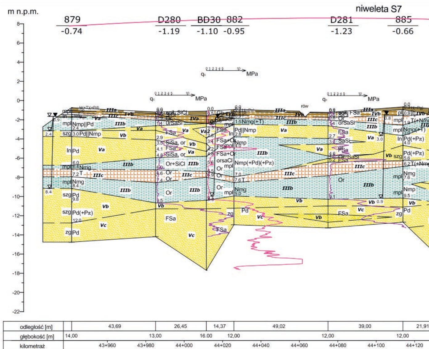
Rys. 1. Typowy przekrój geotechniczny Żuławy Wiślanej (obszar pierwszego poletka próbnego)
