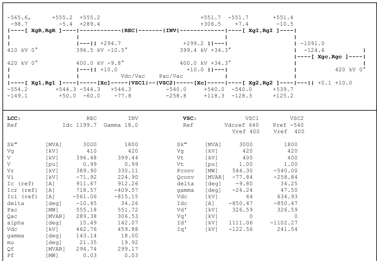
Rys. 4.2 Wyniki rozplwywu mocy dla układu wspólnego LCC-VSC dla modelu nieliniowego
