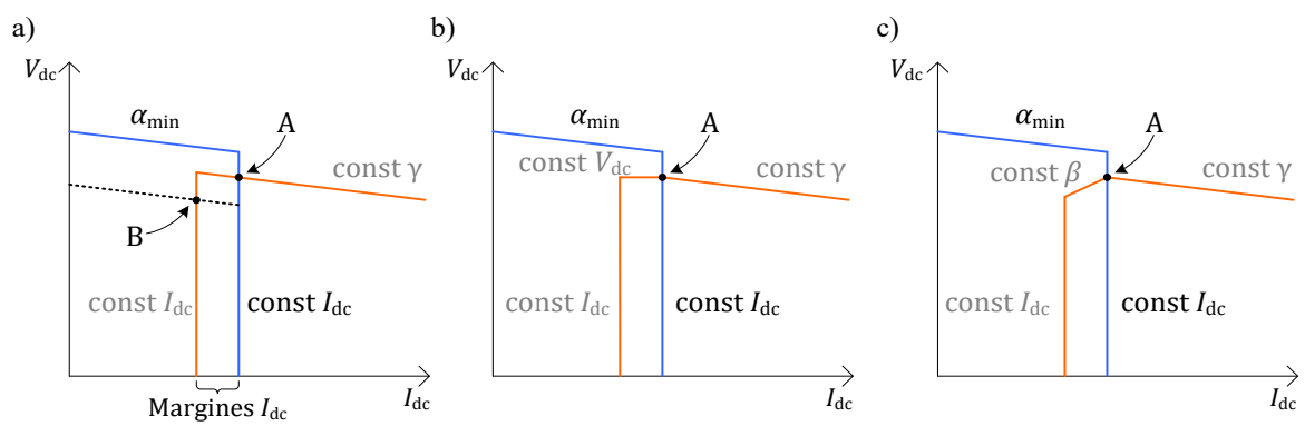
Rys. 2.8 Charakterystyki prądowo-napięciowe prostownika (niebieski) i falownika (pomarańczowy) dla falownika pracującego w trybie: a) regulacji kąta gamma, b) regulacji kąta gamma lub regulacji napięcia DC, c) regulacji kąta gamma lub regulacji kąta beta
