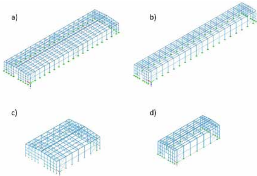
Rys. 1. Geometria czterech analizowanych konstrukcji: a) hala 1, b) hala 2, c) hala 3 oraz d) hala 4
