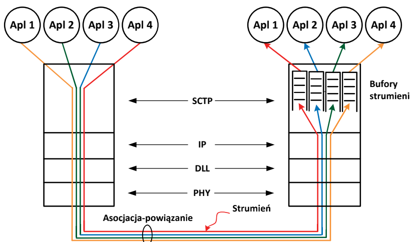
» Rys. 14. Poglądowa ilustracja asocjacji SCTP, strumieni oraz ich obsługi w urządzeniu końcowym (na podstawie: [33])
